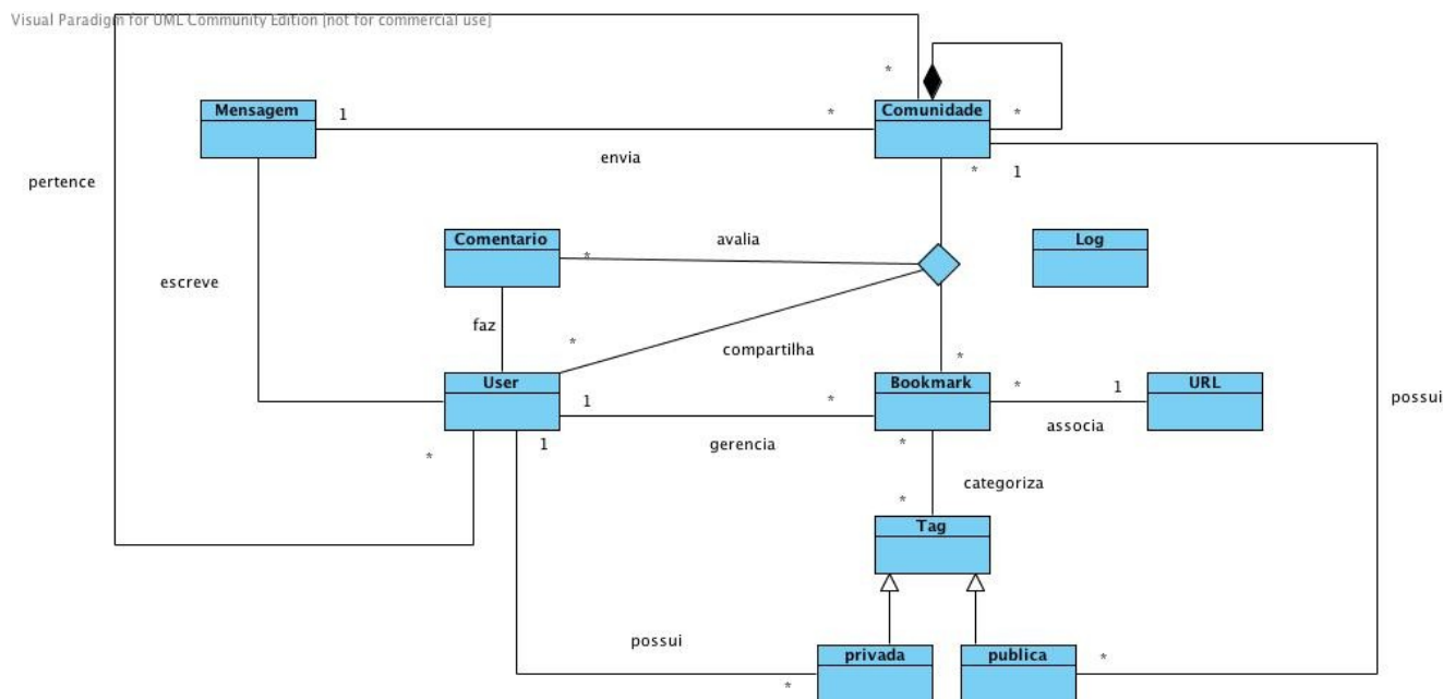
Figura 2: Diagrama de Classe
